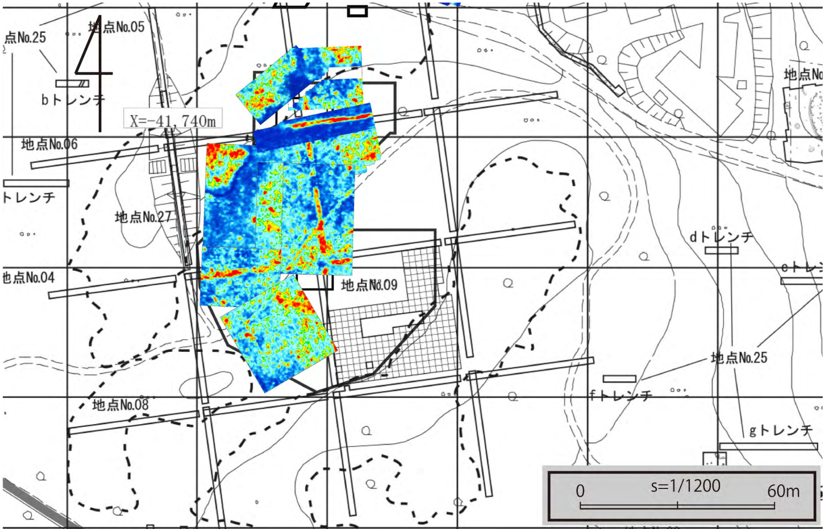
図 1 0 2020 度南貝塚 GPR 地中レーダー探査成果図
