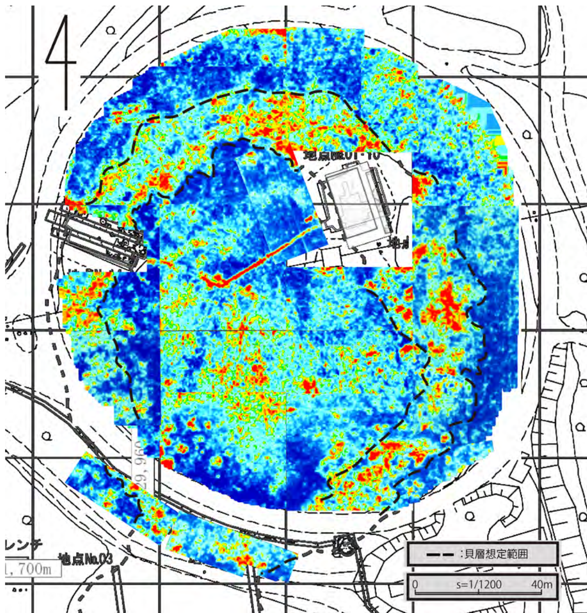
図8 2018年度～2020年度北貝塚 GPR 地中レーダー探査成果図
